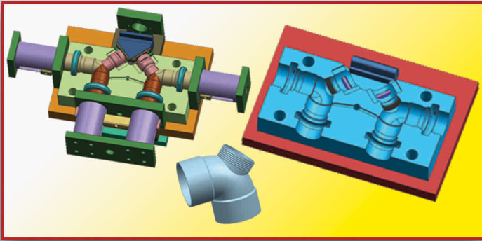
PVC Door Elbow Mould
